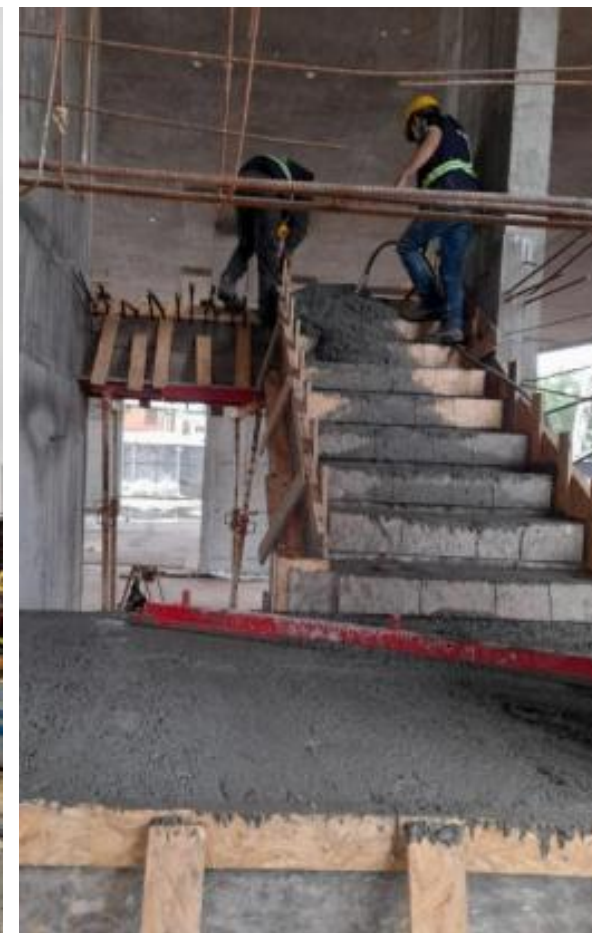
Cargamento Losa N7 – Cargamento de pilares N7 – N8 - Cargamento de escalera PB – N1
