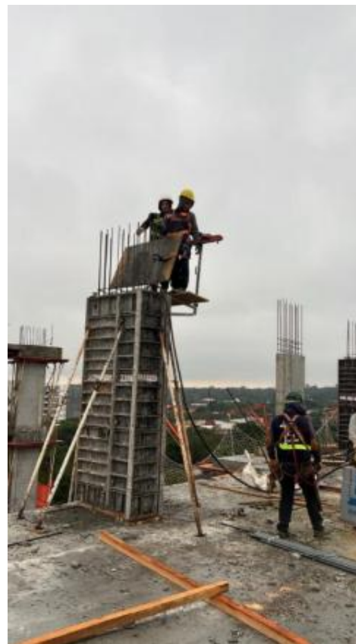
Cargamento Losa N7 – Cargamento de pilares N7 – N8 - Cargamento de escalera PB – N1
